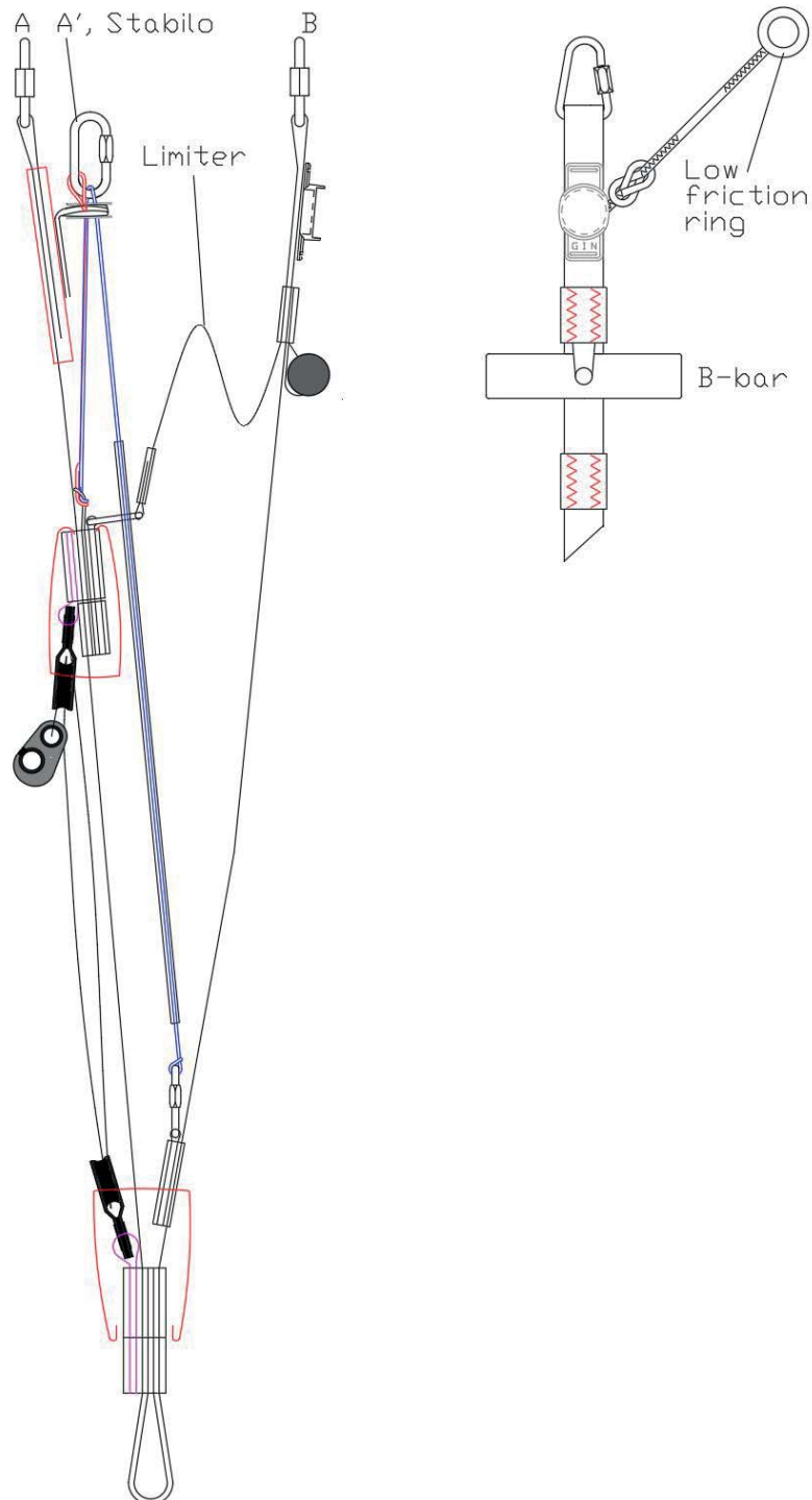
Illustration : élévateurs Bonanza 3
