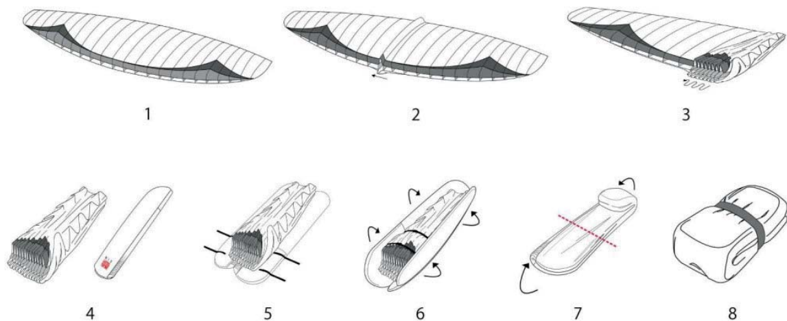
Illustration : plier la Bonanza 3
